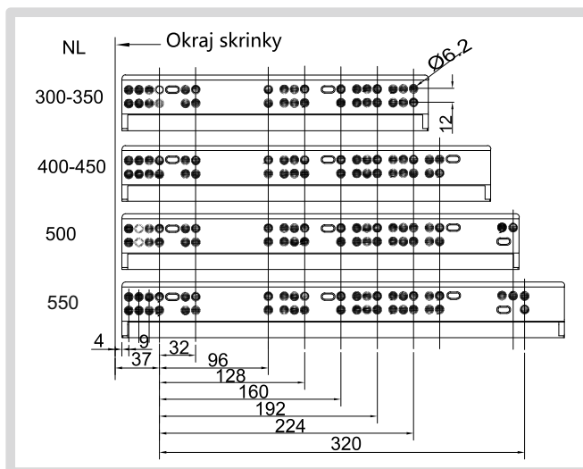
Rozmery pre upevnenie korpusovej lišty
