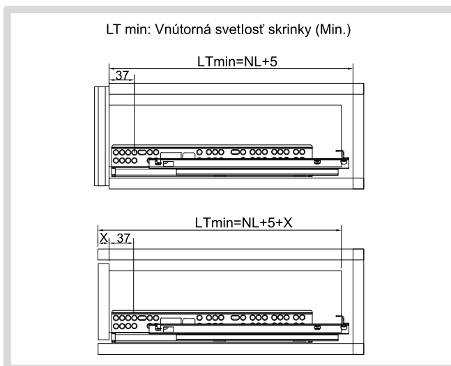
Rozmery pre montáž korpusovej lišty
